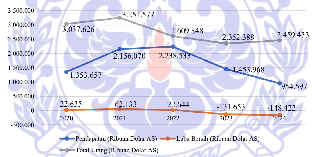
Gambar 1.1 Grafik kinerja keuangan PT Krakatau Steel (Persero) Tbk Tahun 2020–2024
